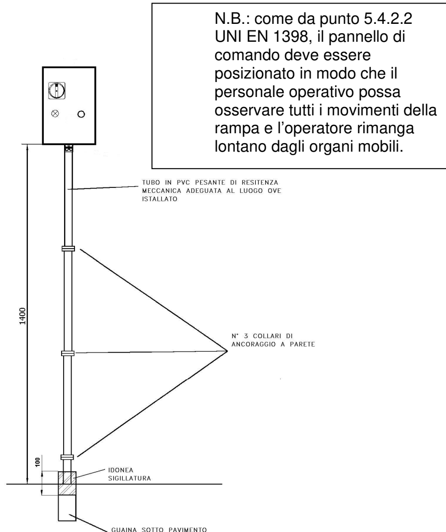
Schema per il collegamento
